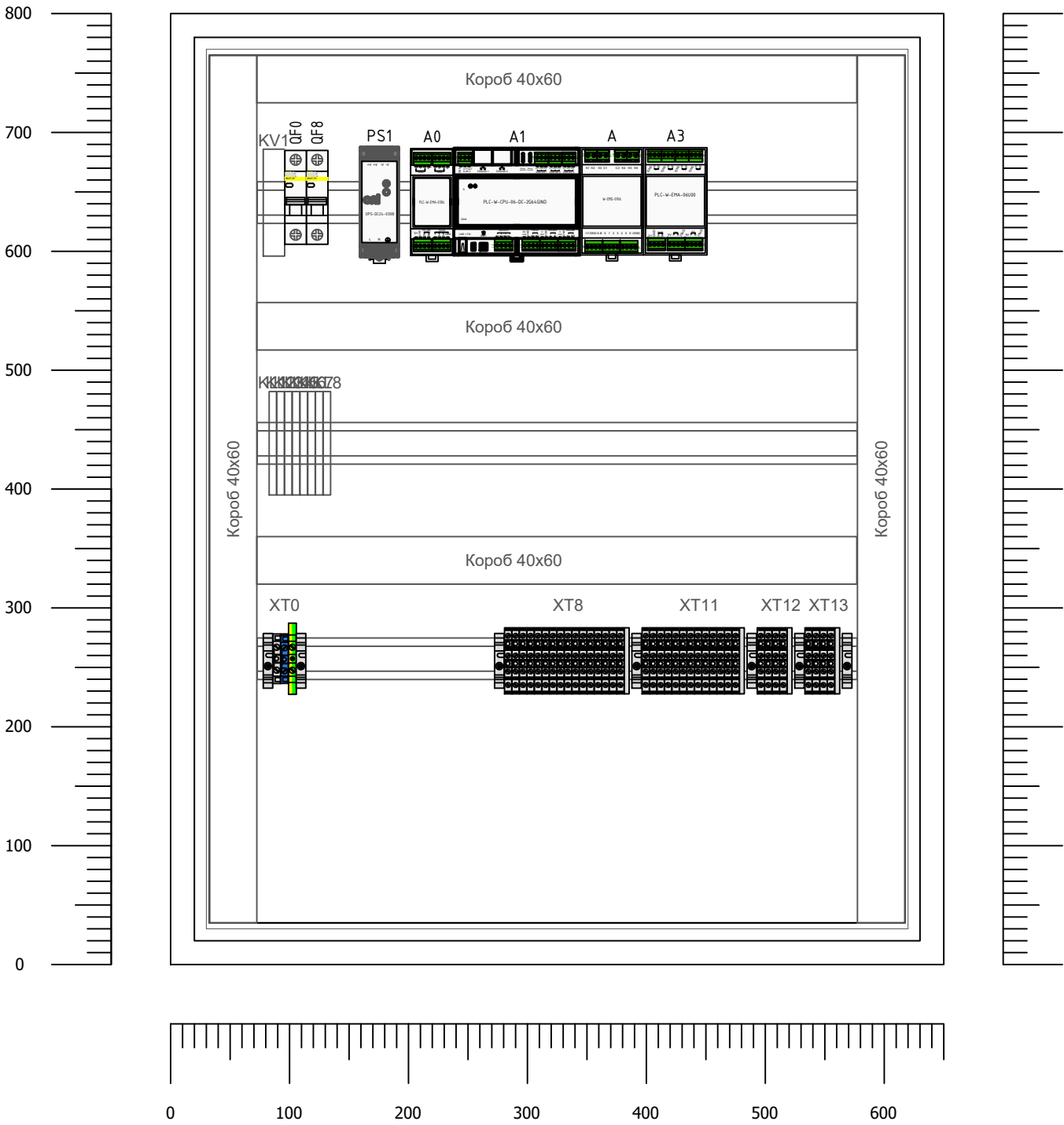
Корпус металлический настенный ЩМП-4-0 36 УХЛ3 IP31 (ШхВхГ) 650x800x250
